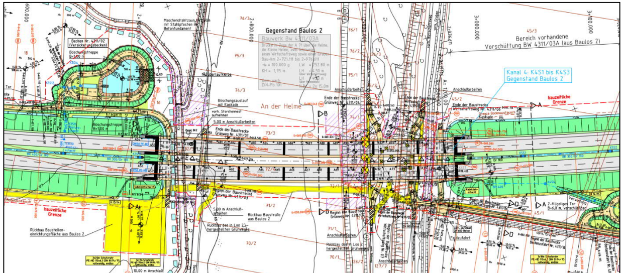
Brücke im Zuge der A 71 über die Helme LW= 252 m (Lageplan)
