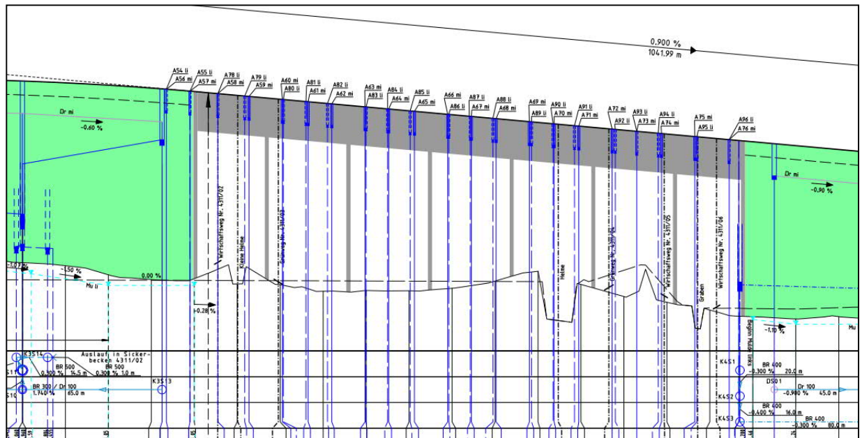
Brücke im Zuge der A 71 über die Helme LW= 252 m (Höhenplan)
