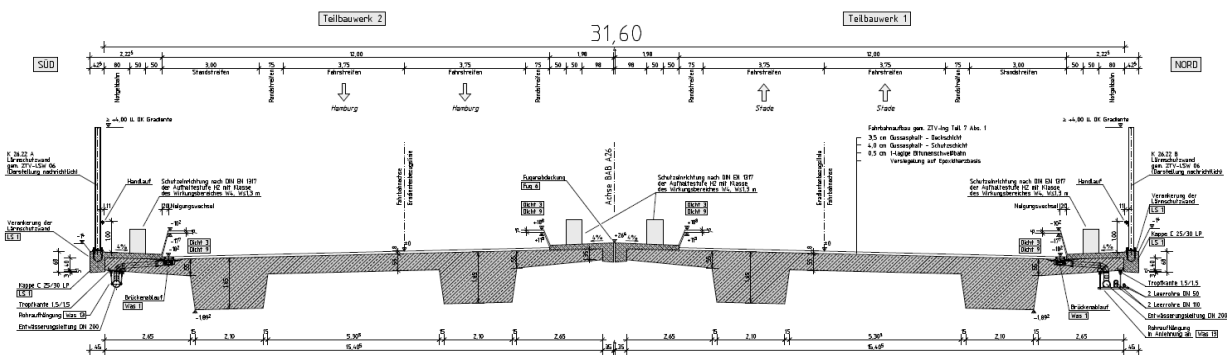
Regelquerschnitt (links: Teil-BW 2 - RiFa Hamburg, rechts: Teil-BW 1 - RiFa Stade)
