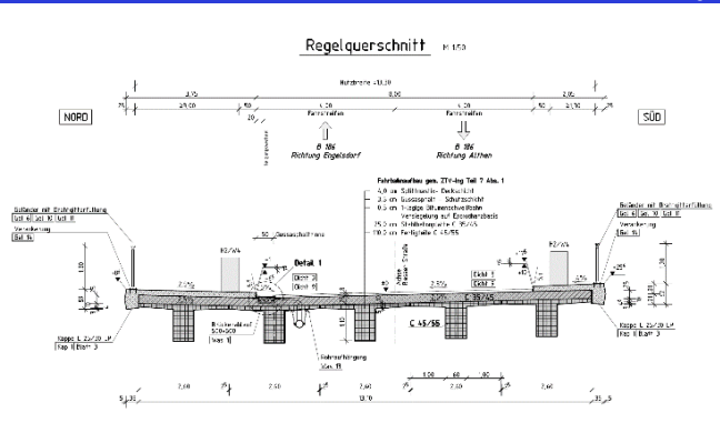
Regelquerschnitt
