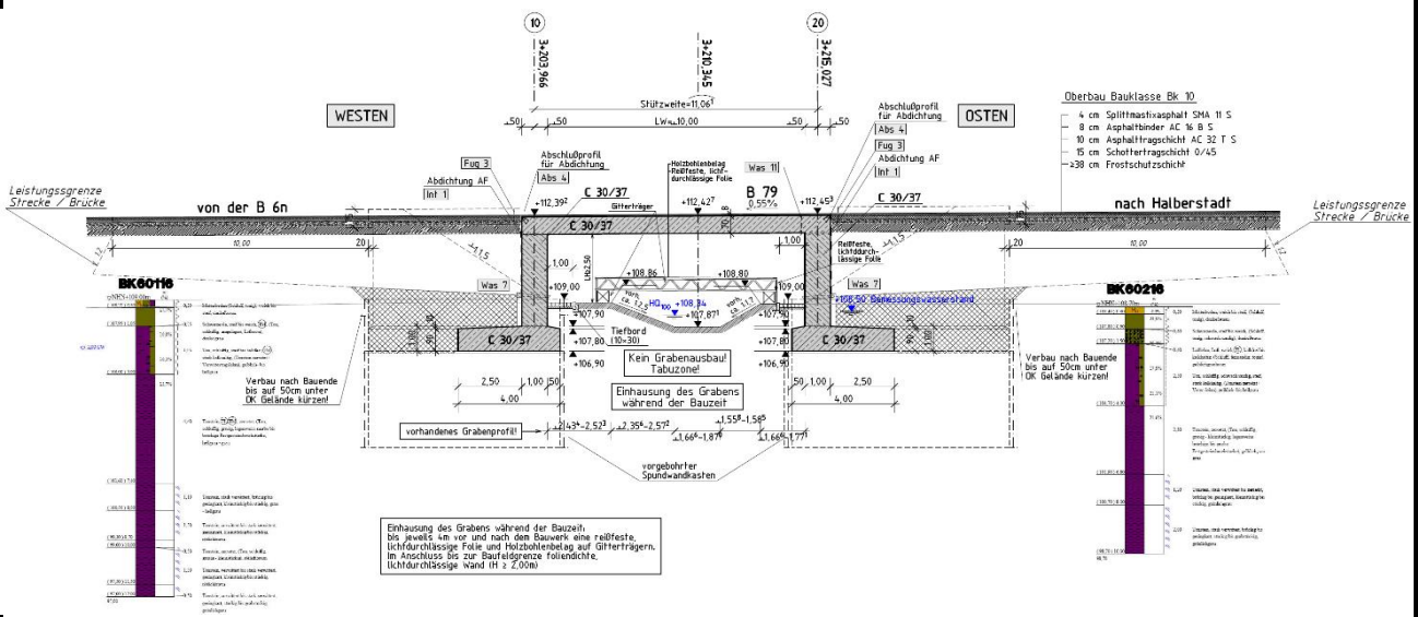
Längsschnitt
